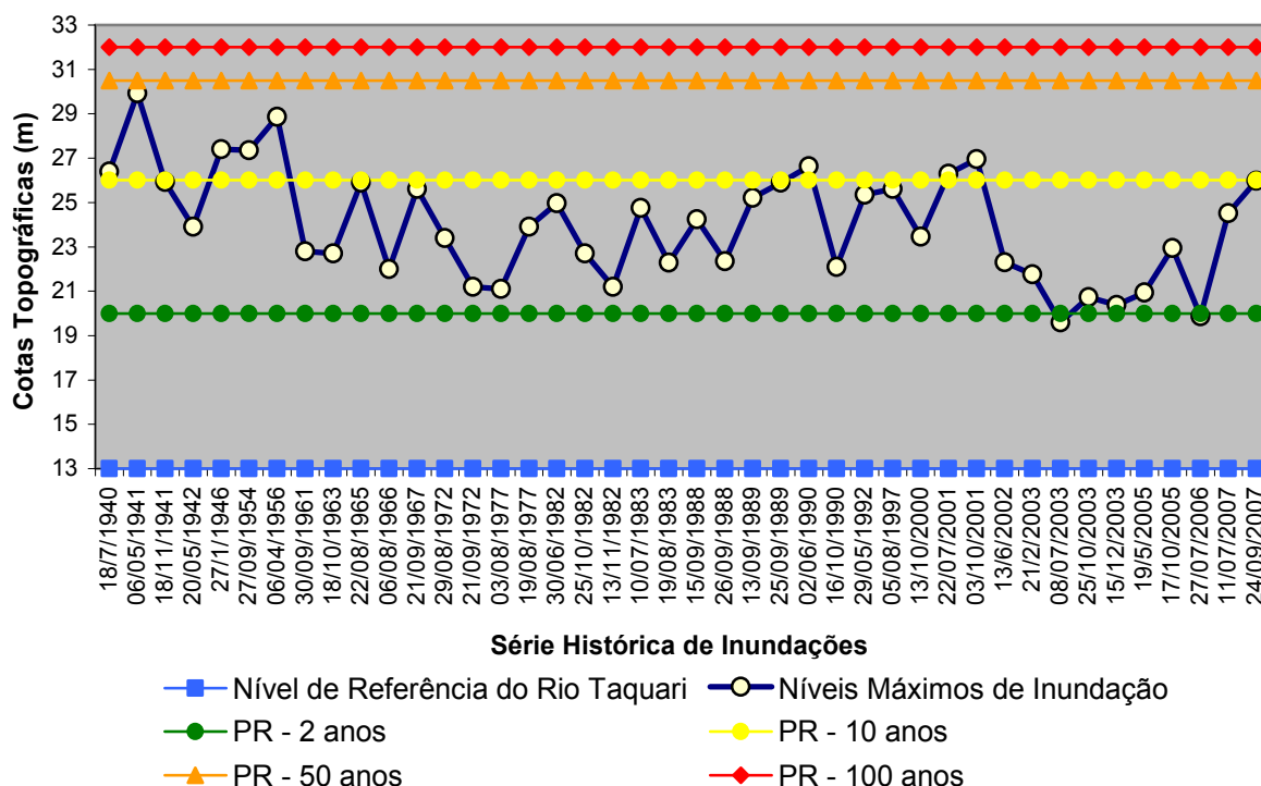
Gráfico 04 - Série histórica dos níveis máximos de inundação acoplada ao período de retorno (PR) calculado para Lajeado
