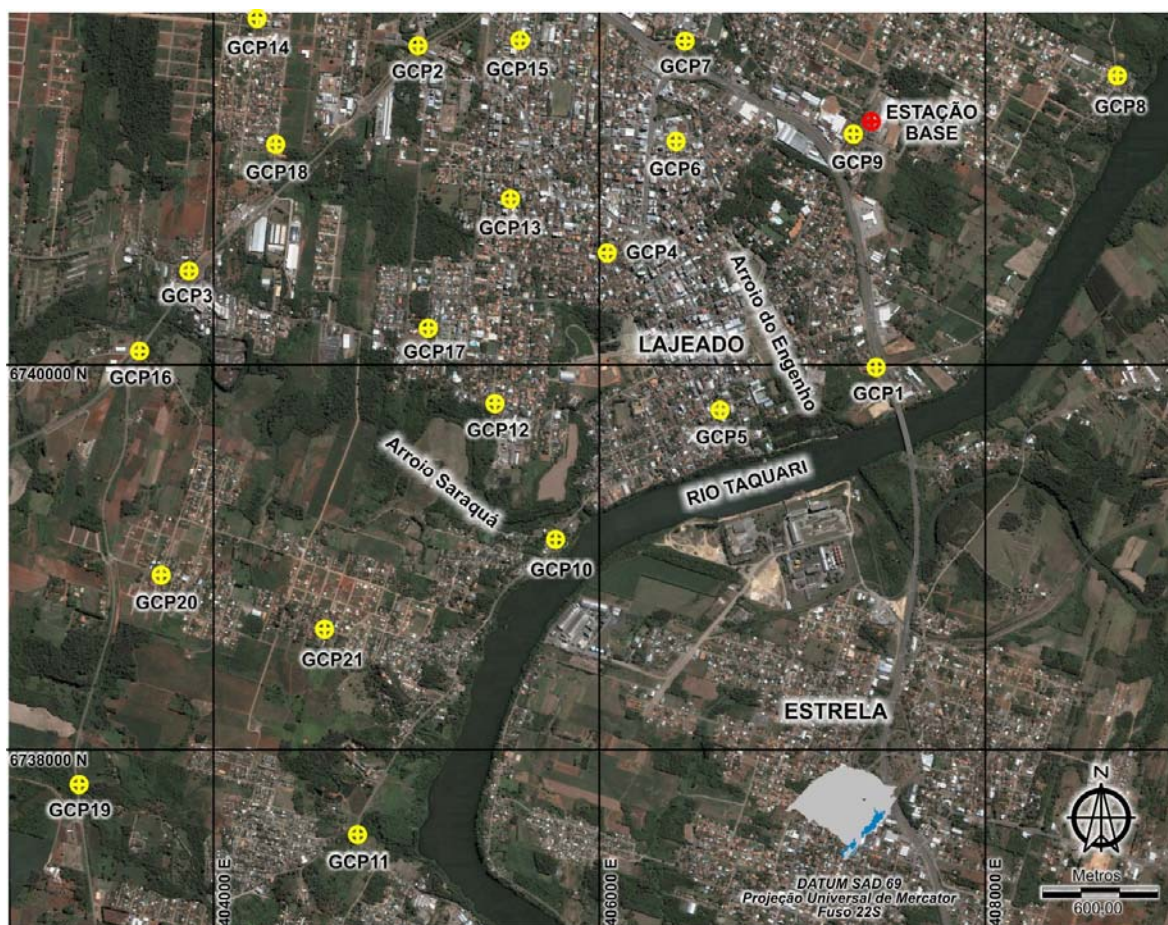
Figura 28 - Distribuição dos GCP e localização da estação-base
