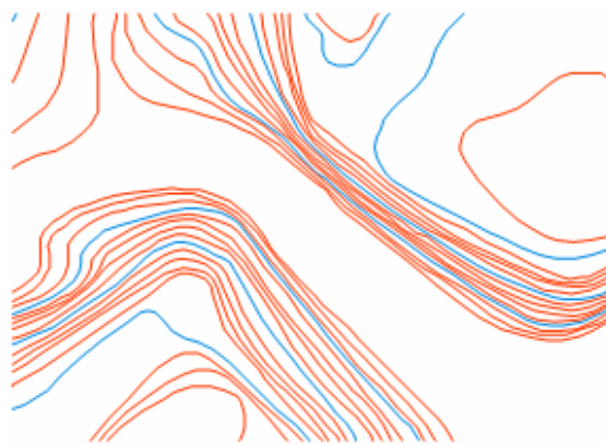
Figura 33 - Digitalização das curvas de nível georreferenciadas
