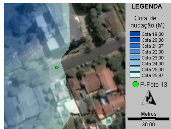
b) Validação da simulação da cota de 25,97 m
