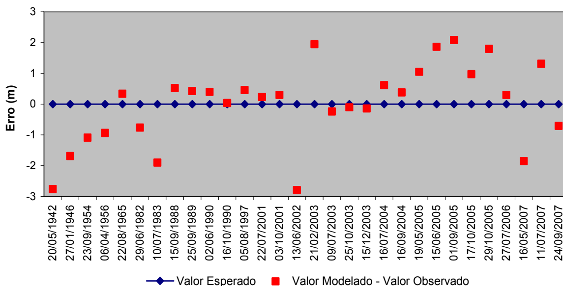
Gráfico 09 - Ajuste dos valores modelados em relação aos valores esperados
