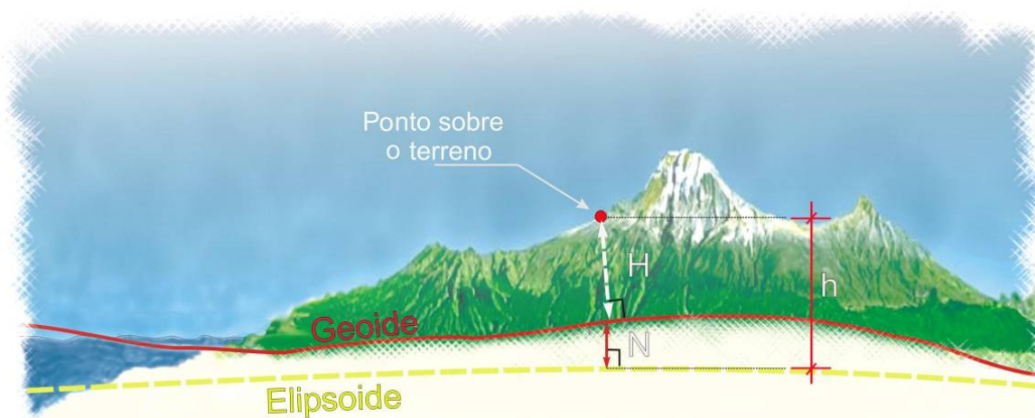
Figura 31 - Esquematização da relação entre o elipsóide e do geóide da Terra
